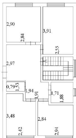
План второго этажа
