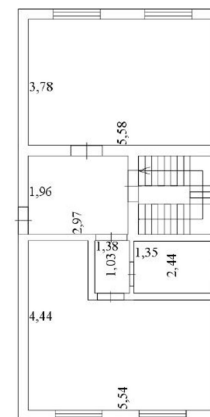
План первого этажа
